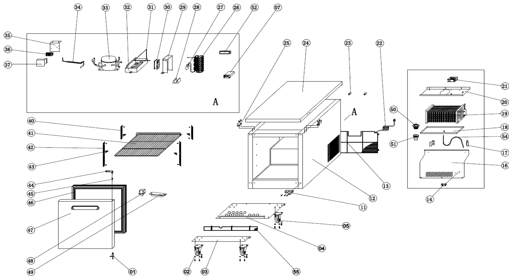
EXPLODE OF HC-TUC27S-32/M38
